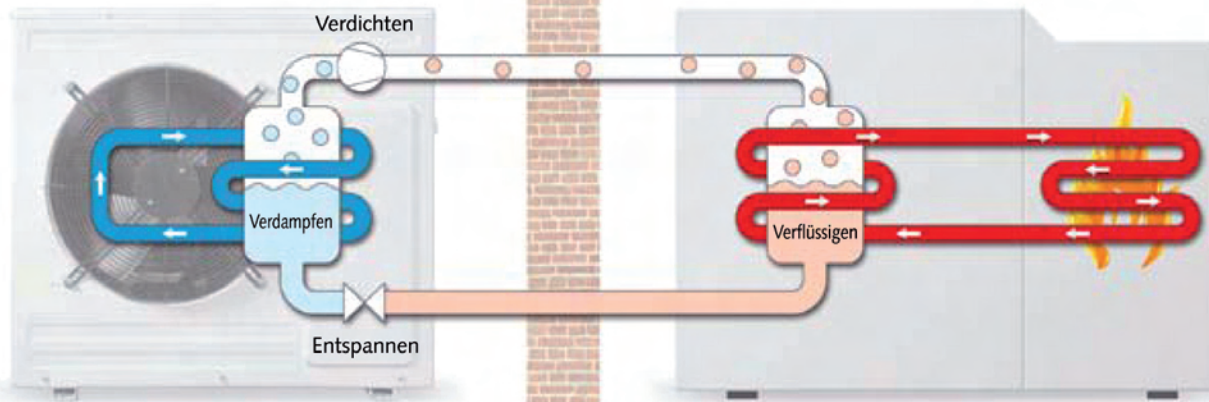
Außenmodul Wärmepumpe
